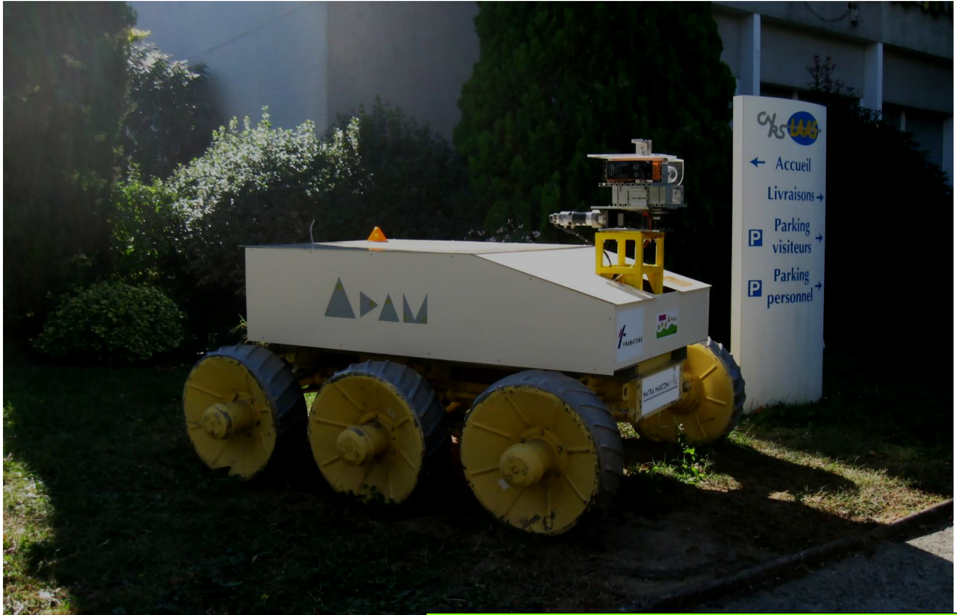
Restauration du Robot d'Exploration Planétaire ADAM Pour le compte du LAAS.
